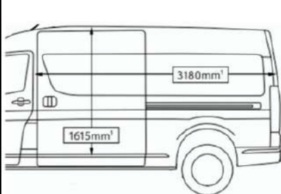
SLWB Bus & Panel Van
